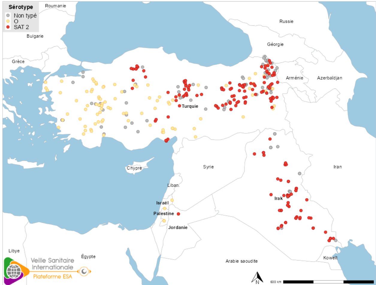
Figure 1. Localisation des foyers de fièvre aphteuse au Proche Orient depuis le 01/01/2023 (source : Commission européenne ADIS le 04/09/2023 et WAHIS-OMSA le 01/09/2023).
